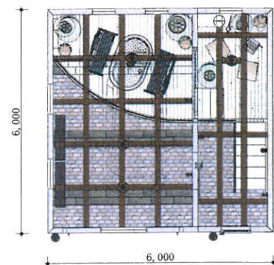
平面図 S=1/100
