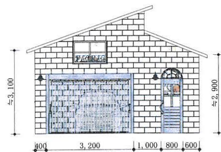
立面図 S=1/100
