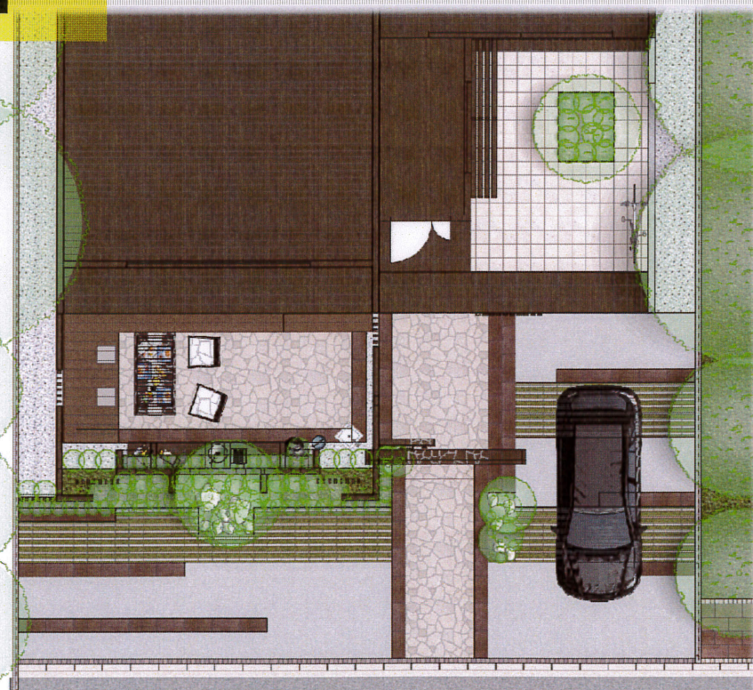
平面図S=1:100
